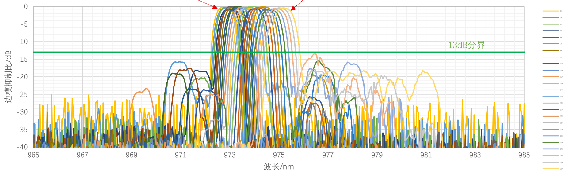
光谱/A
